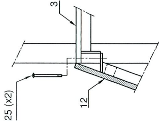
Détail 2 - Assemblage du mur d'escalade sur la tour A.
